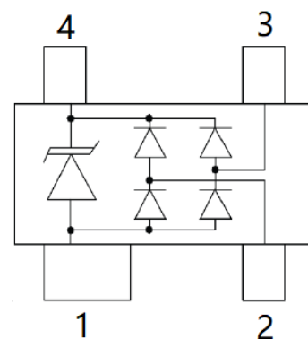
SOT-143
